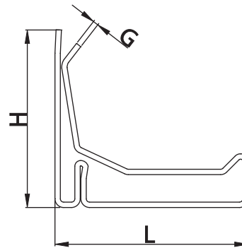
Profil PQ-C
